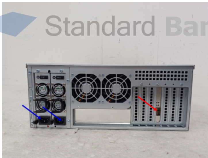
제품 포트 #2
