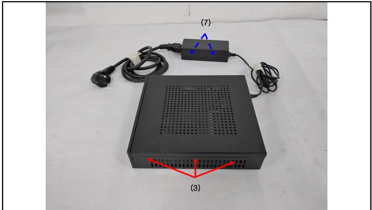
제품 좌측면
