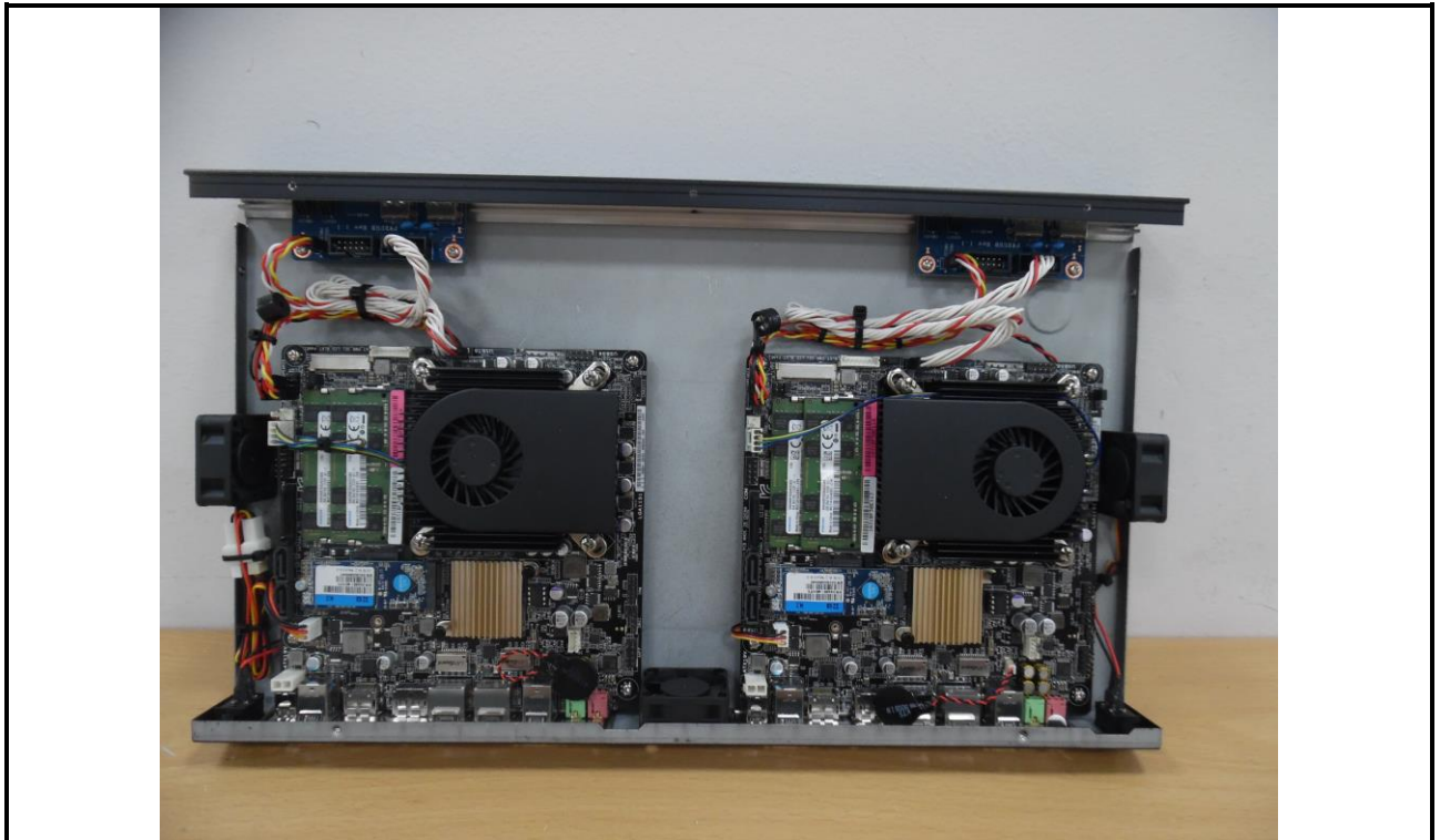
제품 내부
