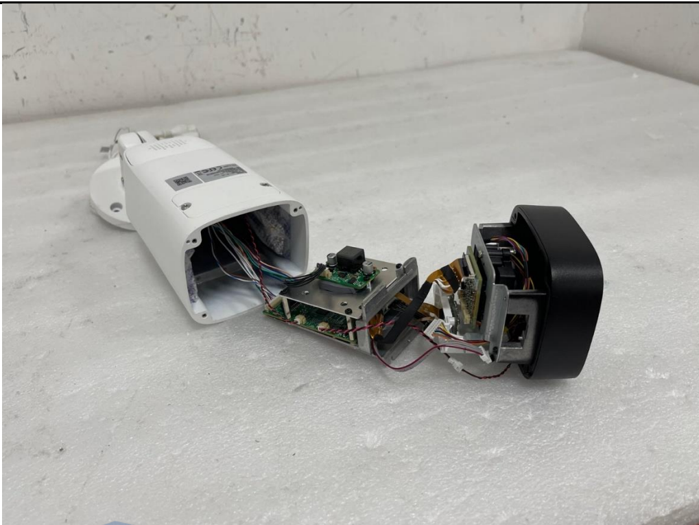
제품 내부
