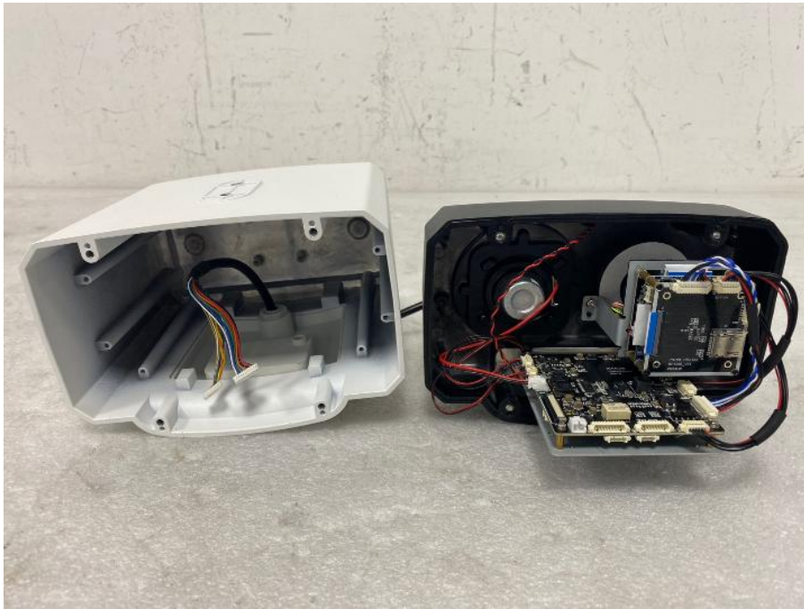
제품 내부
